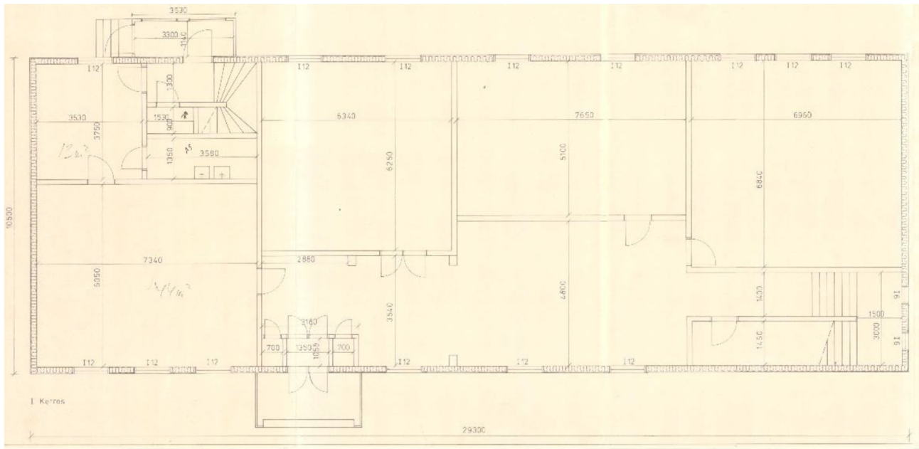
Kuva 1. 1. kerroksen pohjapiirros © Osmo Heikkilä, 1984
