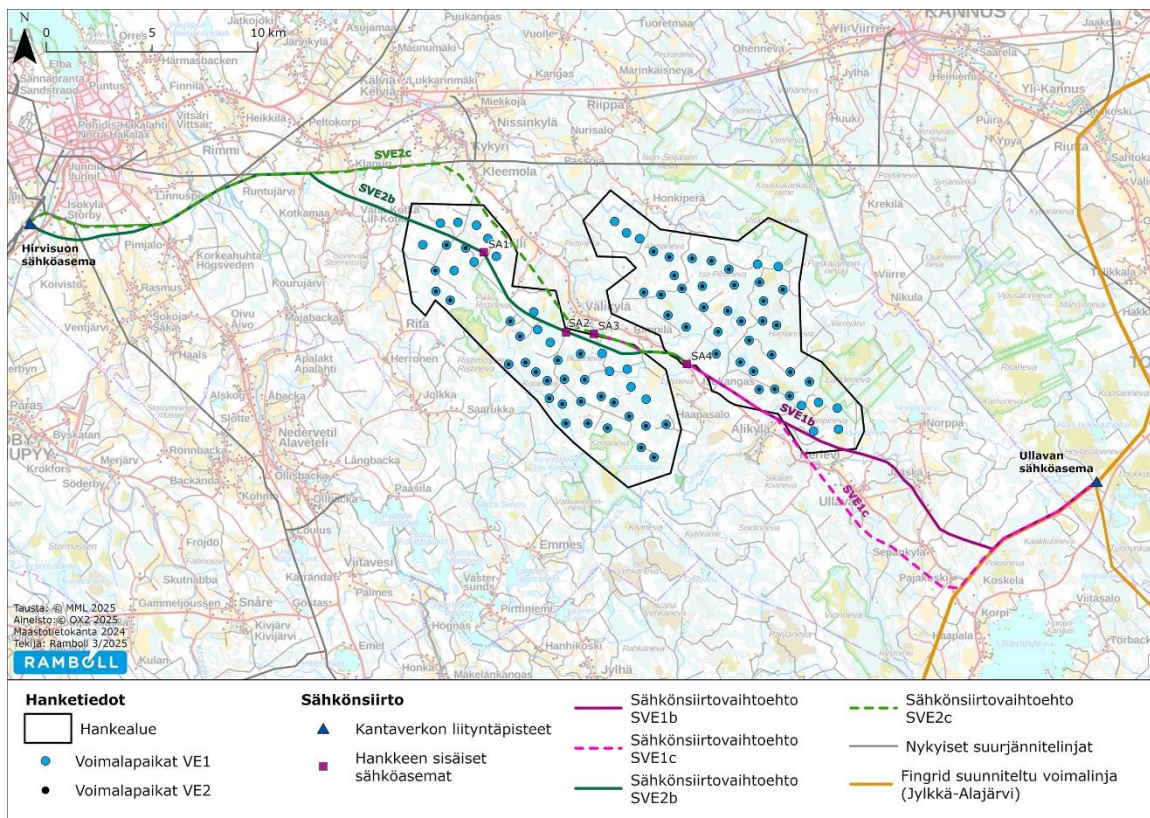
Kuva 1. Pihtinevan tuulivoimahankkeen hankealue, vaihtoehdot VE1 (86 tuulivoimalaa) ja VE2 (60 tuulivoimalaa), sähköasemien vaihtoehdot (SA1-SA4) sekä sähkönsiirtoreittien vaihtoehdot SVE1b, SVE1c, SVE2b ja SVE2c.
