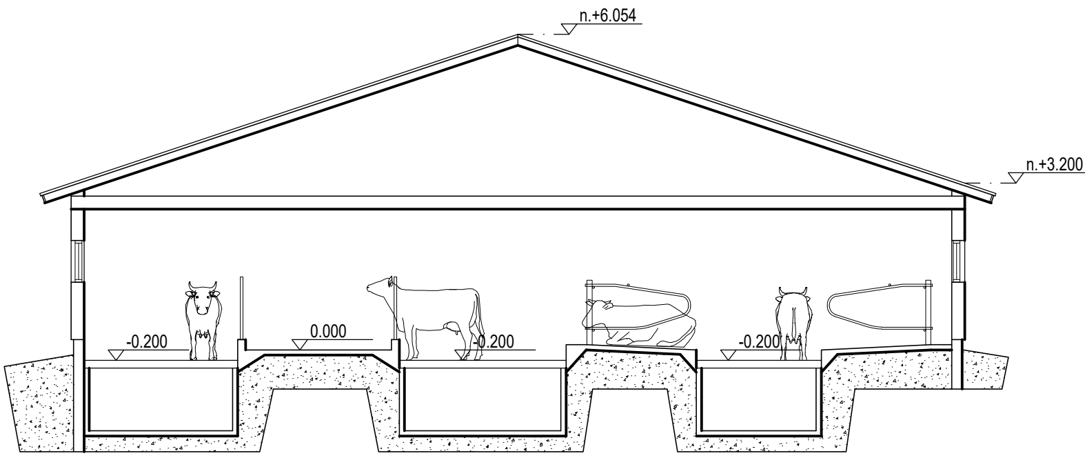
LEIKKAUS A - A
