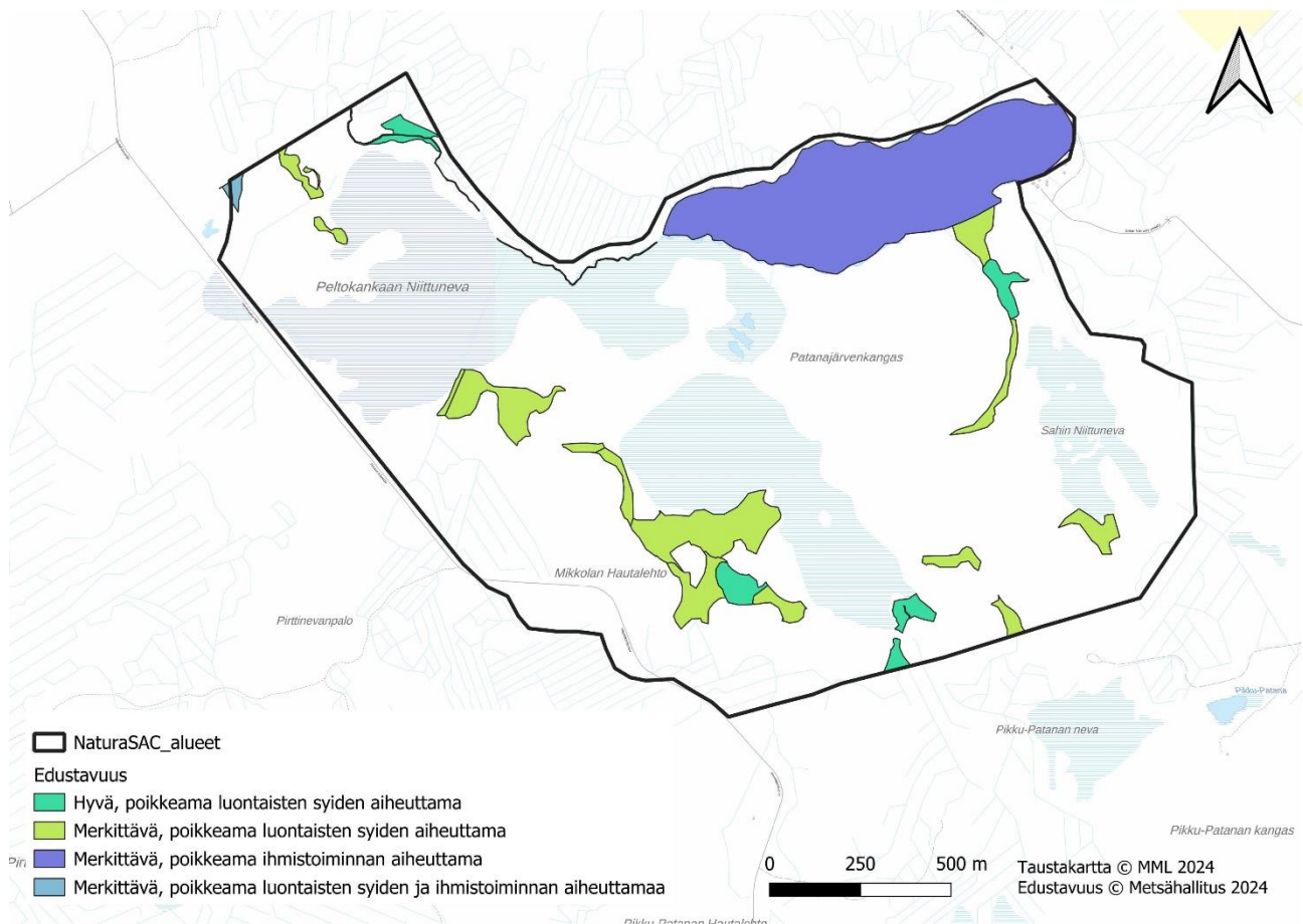
Kuva 4. Naturaluontotyyppien edustavuus. Tyhjiille alueille edustavuutta ei ole määritetty.
