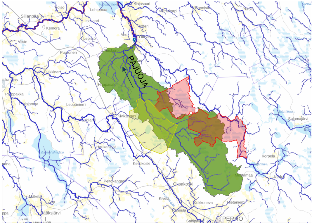
Kuva 3. Pajuoja valuma-alue. Pajuoja laskee luoteeseen kohti Penninkiojaa. Hankealue on esitetty kuvassa keltaisella ja Natura-alue punaisella värillä. Valuma-alue on tarkasteltu Scalgo Live -työkalun avulla.
