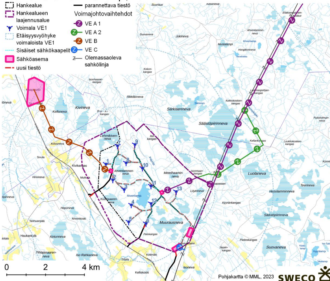
Kuva 2. Voimalasijoittelu vaihtoehdossa VE1 ja hankkeen sähkönsiirtovaihtoehdot.
